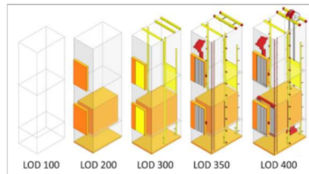
Gambar 2 Level of Detail pada BIM
