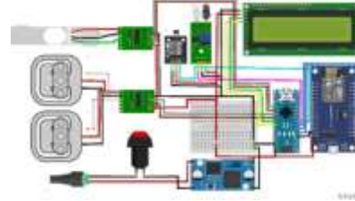
Gambar 1. Rangkaian Instrumentasi Dinamometer Berikut merupakan keterangan pengkabelan komponen yang digunakan:
